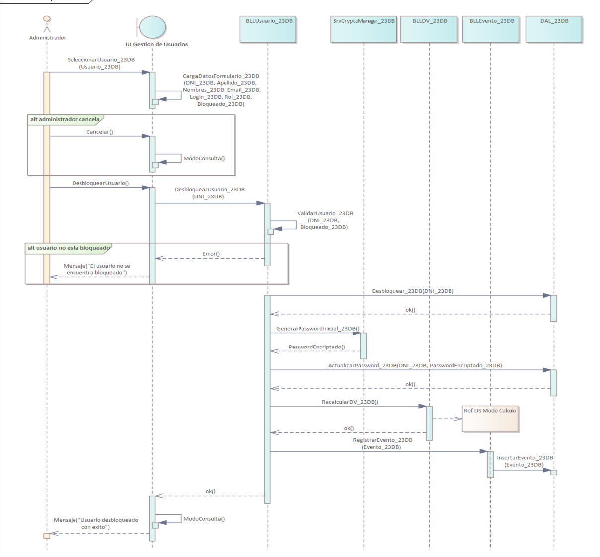
sd D503 - Desbloquear Usuario
