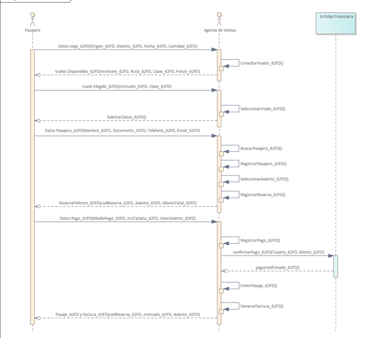
sd Diagrama de Secuencia de Roles
