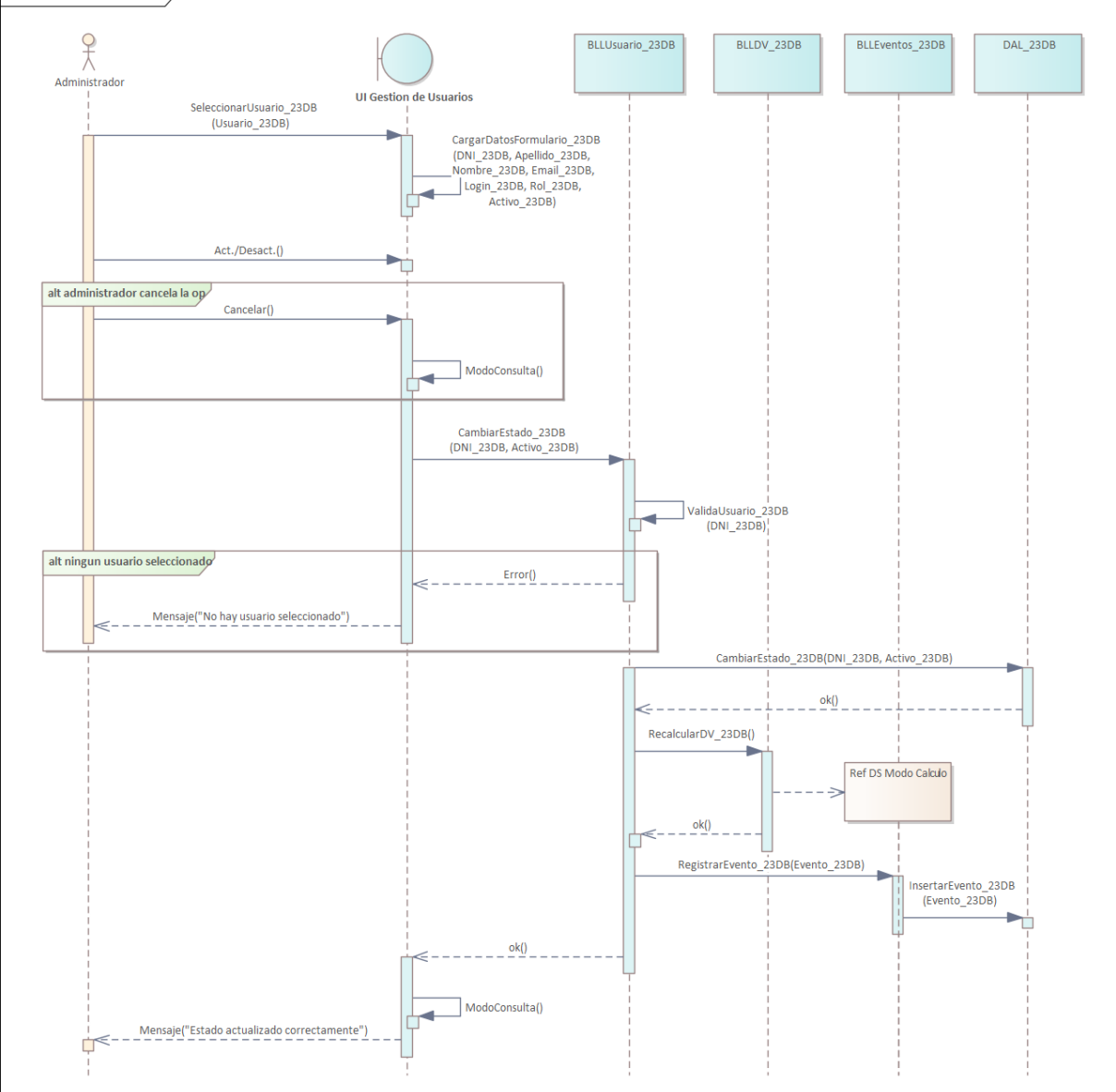
sd D507 - Act./Desact. Usuario
