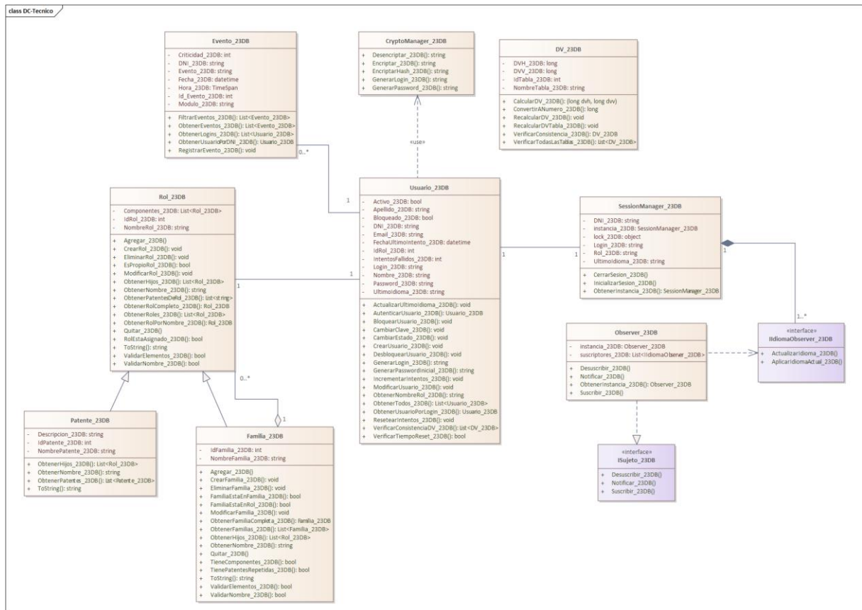
Diagrama de Clases General por Capas
